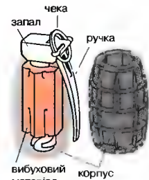
Ручна граната
